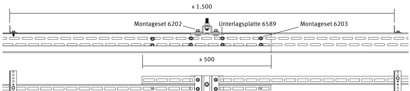
Profilstoß: Einfachträger C- oder UA-Profile im Bereich einer Abhängung oder Befestigung, Profile Rücken an Rücken um 500 mm versetzt miteinander mit Montageset 6203 verschraubt
